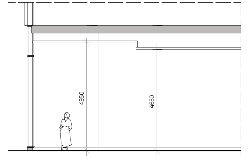
SEKTION
